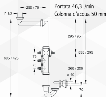
3) Collettore orizzontale idoneo per distanze molto limitate fra piletta e punto di scarico
