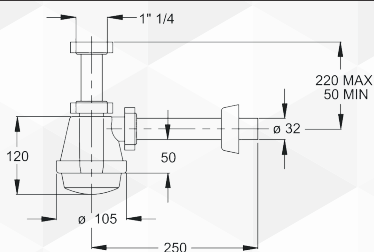
0479402 Portata 46,6 l/min Colonna d'acqua 50 mm
