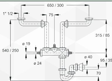
Portata 46,3 l/min Colonna d'acqua 50 mm
