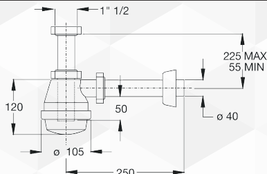
0479404 Portata 65 l/min Colonna d'acqua 50 mm
