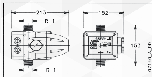
Scheda elettronica per GENYO 16 A
