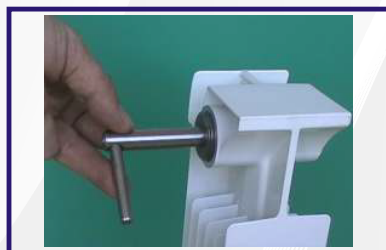
1: Inserimento della fresa di pulizia della filettatura nel mozzo del radiatore.
