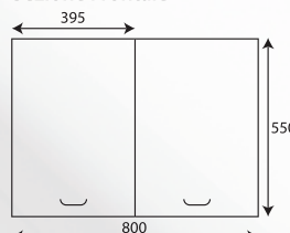
Sezione Frontale
