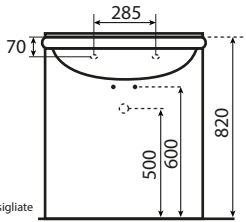
Misure di ingombro per mobile
