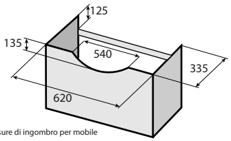
Misure di ingombro per mobile
