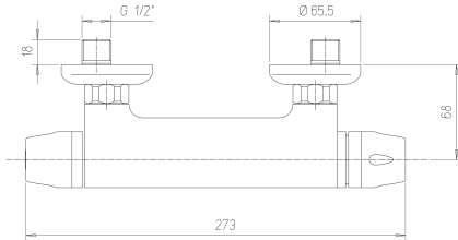
CARTUCCIA TERMOSTATICA 04224
