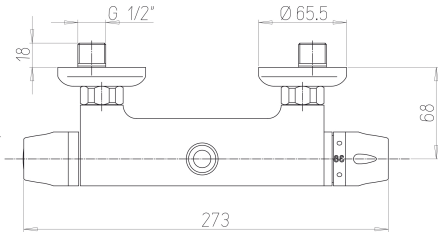
CARTUCCIA TERMOSTATICA 04224
