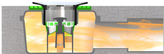
Valvola antiodore in posizione normalmente chiusa
