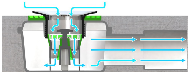
Valvola antiodore in posizione aperta
