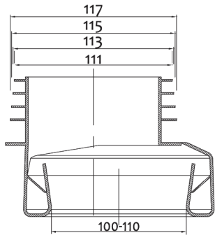
SEZIONE A-A SECTION A-A
