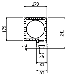
ATTACCO LATERALE*
