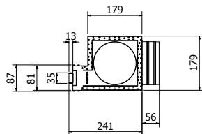
ATTACCO POSTERIORE
