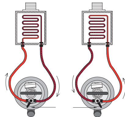
Abb. 1 - Strömungsrichtung im Uhrzeigersinn Abb. 2 - Strömungsrichtung gegen den Uhrzeigersinn
