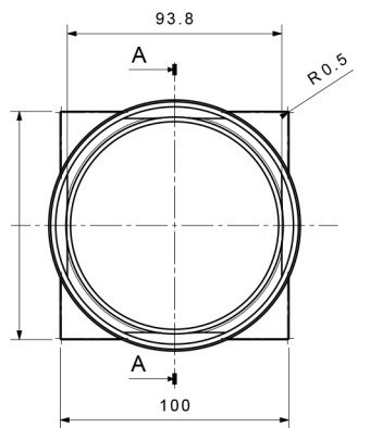
Bottom view Scale: 1:2
